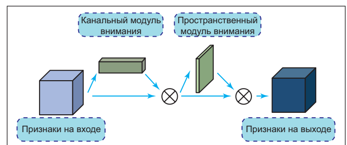
Рис. 5. Архитектура алгоритма обнаружения дефектов
